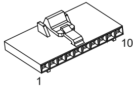
Sicht auf die Buchsenseite
